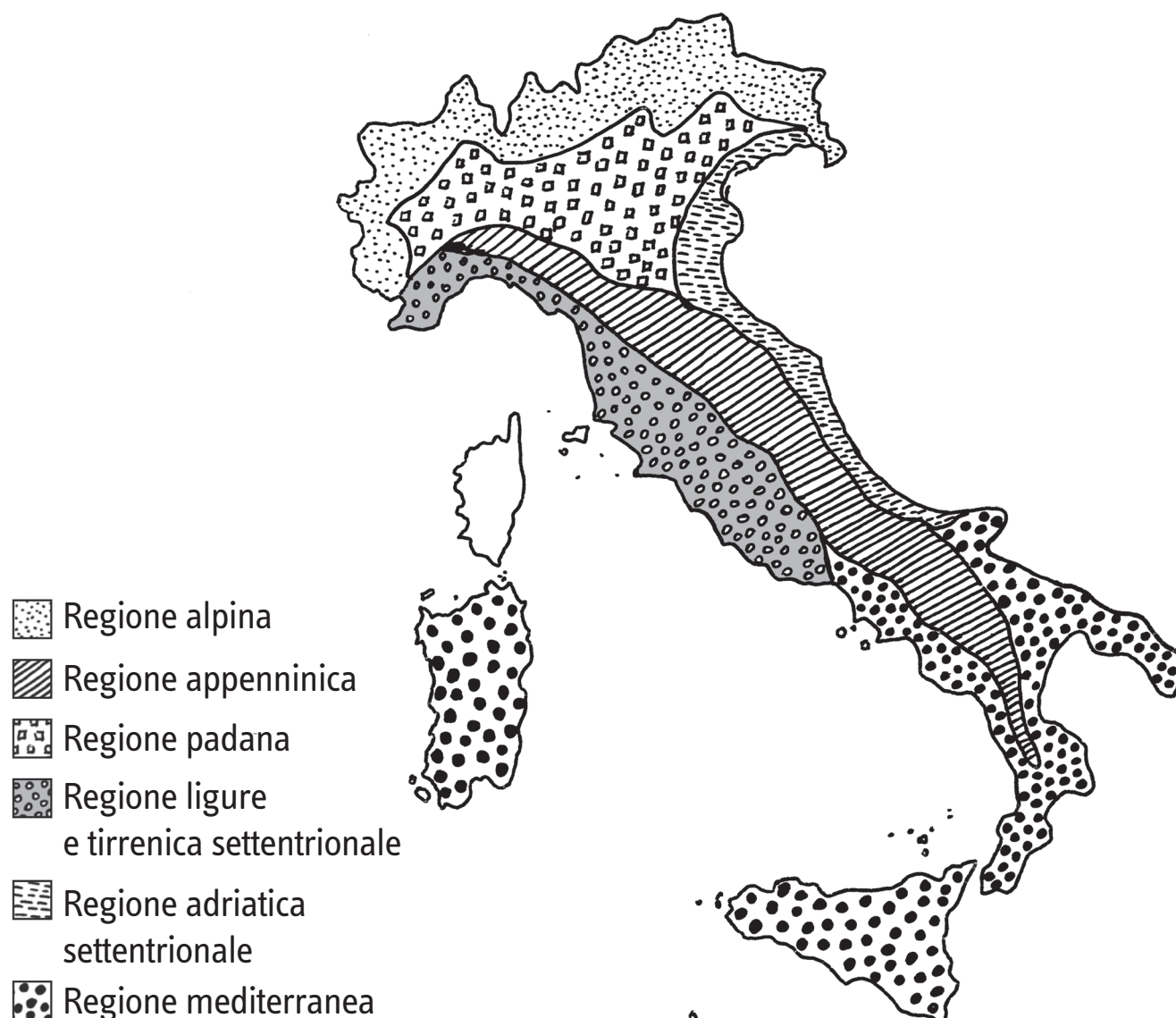
FIGURA 4. Carta tematica delle principali regioni climatiche italiane
