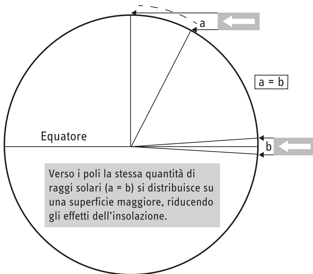
FIGURA 3. Rappresentazione schematica della diversa inclinazione dei raggi solari e della differente intensità di insolazione sulla superficie terrestre
