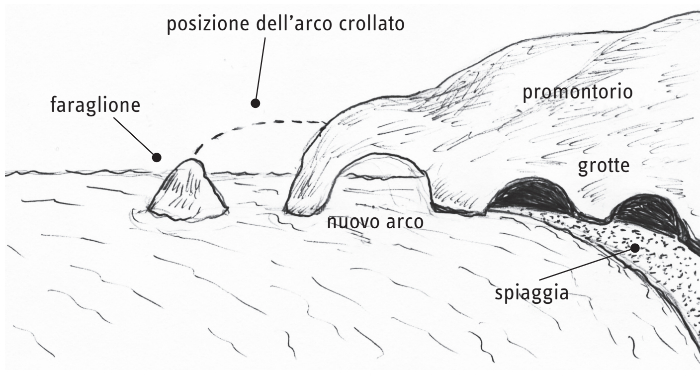
FIGURA 18. Schema della formazione dei faraglioni nella costa alta e rocciosa
