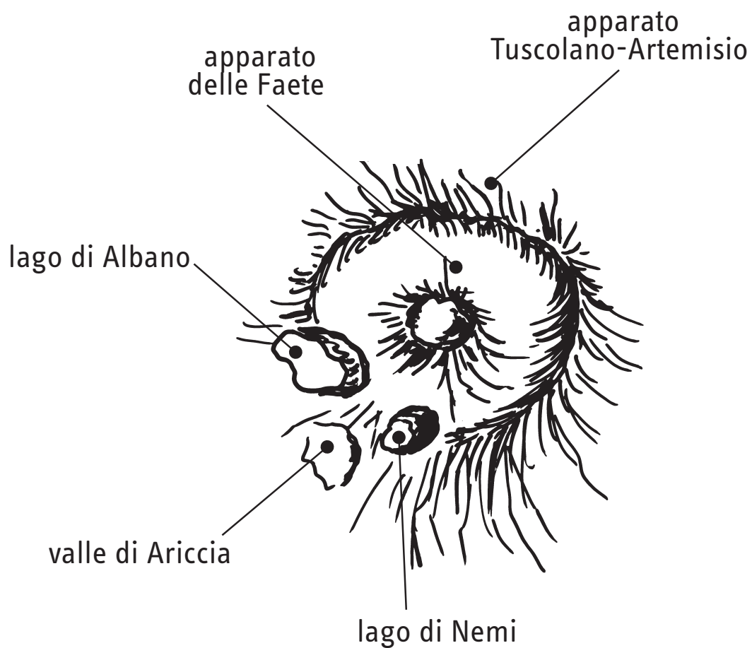
FIGURA 15. Schematizzazione dell'apparato del Vulcano Laziale
